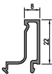
Junquillo 8 mm 40508
