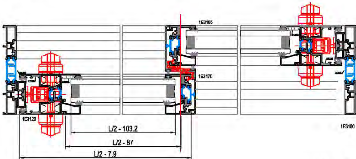
Escala Sección 1:3
