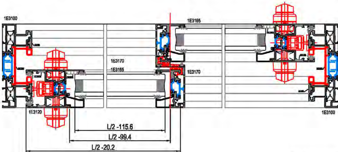
Escala Sección 1:3
