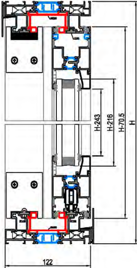
Escala Sección 1:3
