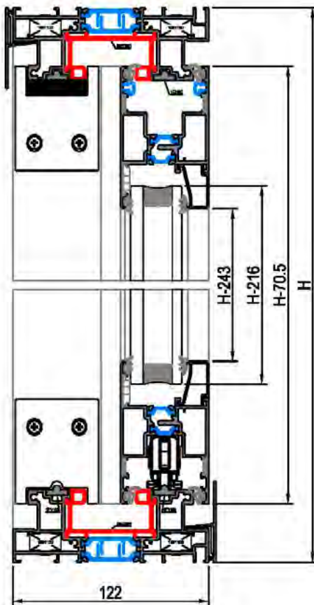
Escala Sección 1:3
