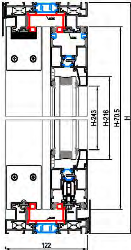
Escala Sección 1:3
