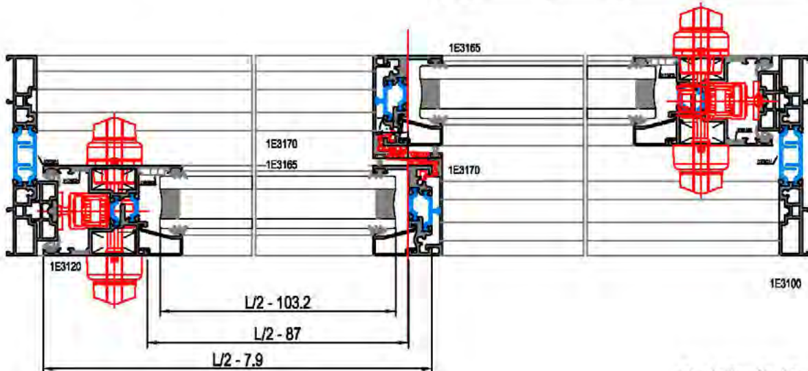
Escala Sección 1:3
