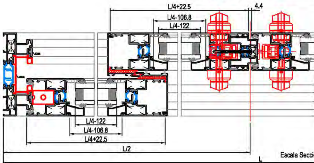
Escala Sección 1:3
