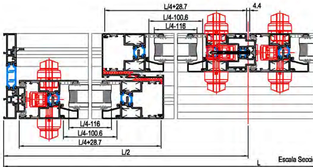
Escala Sección 1:3
