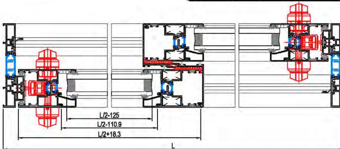
Escala Sección 1:3
