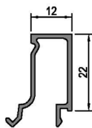
Junquillo 12 mm 40512
