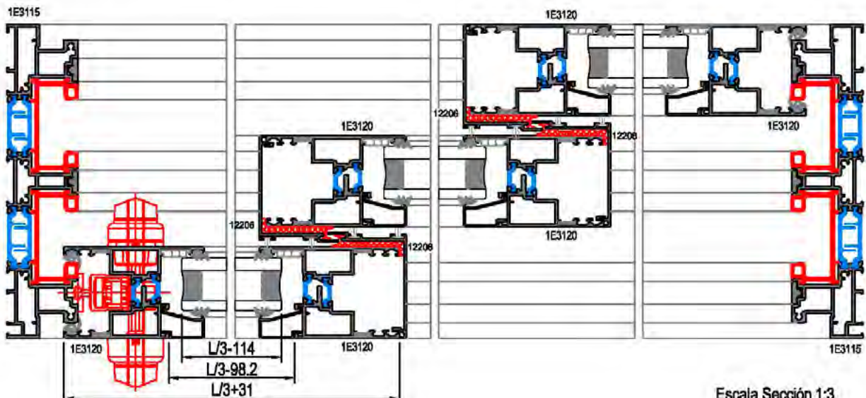
Escala Sección 1:3
