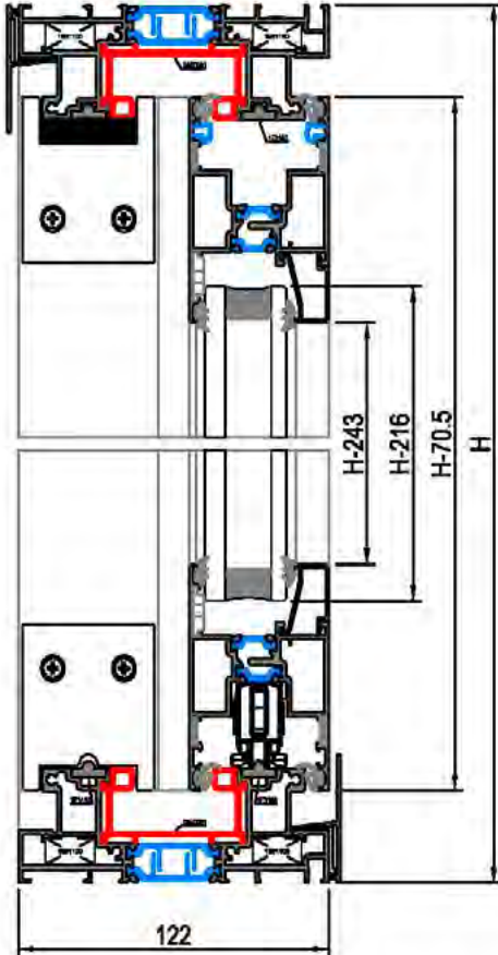
Escala Sección 1:3
