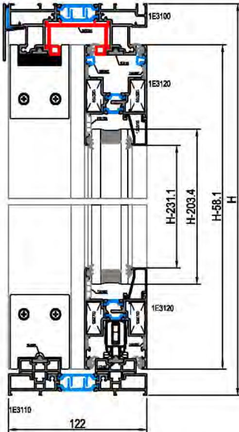
Escala Sección 1:3
