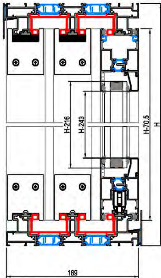
Escala Sección 1:3
