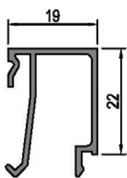
Junquillo 19 mm 40519
