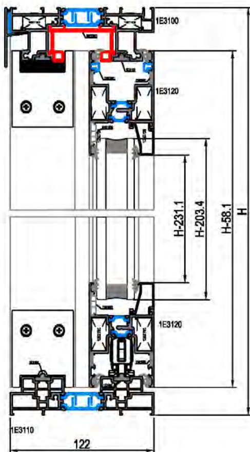
Escala Sección 1:3
