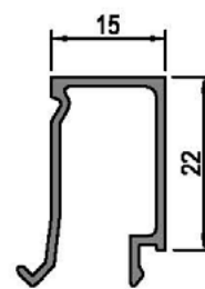
Junquillo 15 mm 40515
