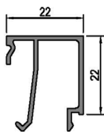
Junquillo 22 mm 40522
