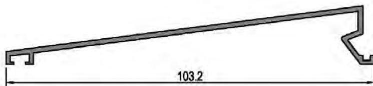
Vierteaguas 100 mm 40082
