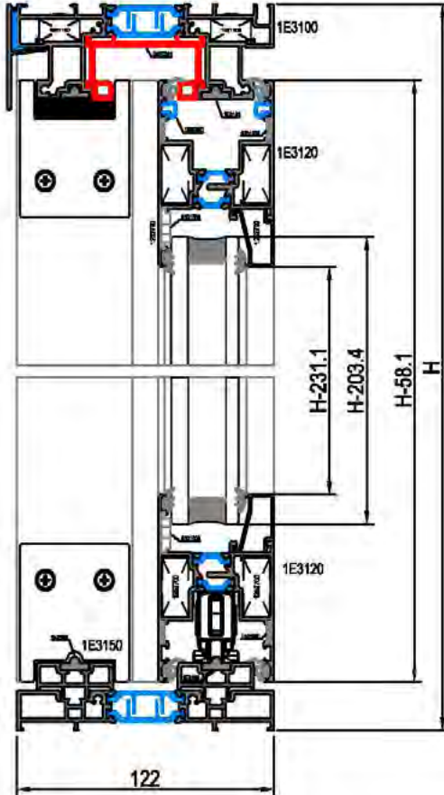
Escala Sección 1:3
