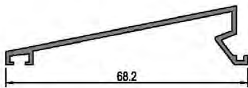
Vierteaguas 68.2 mm 0122
