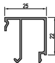
Junquillo 25 mm 40525
