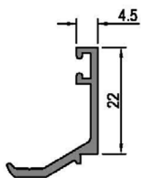
Junquillo 4,5 mm 40505
