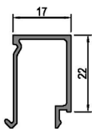
Junquillo 17 mm 40517
