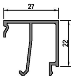
Junquillo 27 mm 40527
