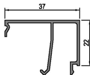
Junquillo 37 mm 40537
